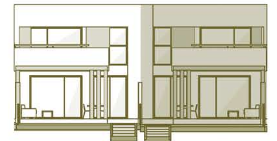
ALZADO
